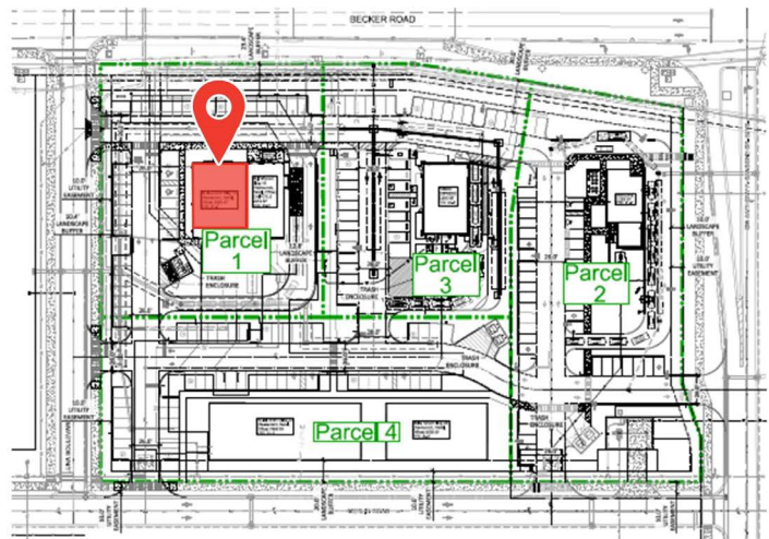
Parcel Plan
