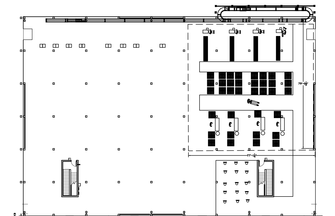
ETAGE - NIVEAU 2 (WALK PICK) MEZZANINE - LEVEL 2 (WALK PICK)
