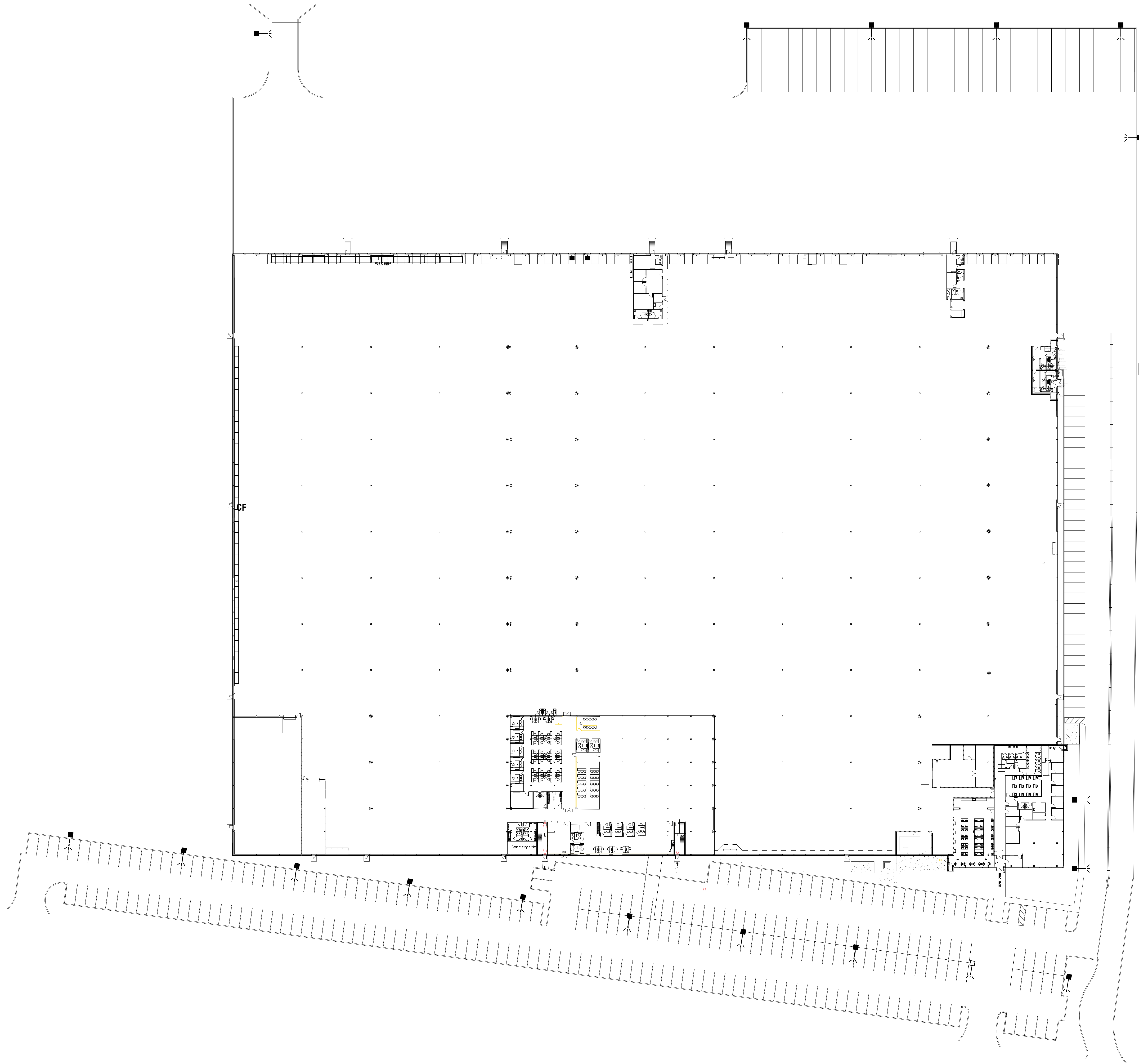
ETAGE - NIVEAU 3 (WALK PICK) MEZZANINE - LEVEL 3 (WALK PICK)
