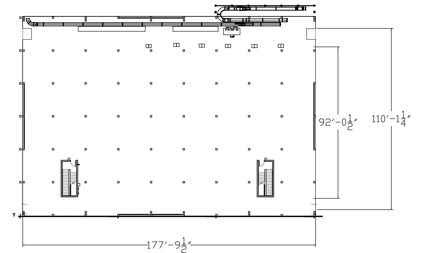
ETAGE - NIVEAU 2 (WALK PICK) MEZZANINE - LEVEL 2 (WALK PICK)
