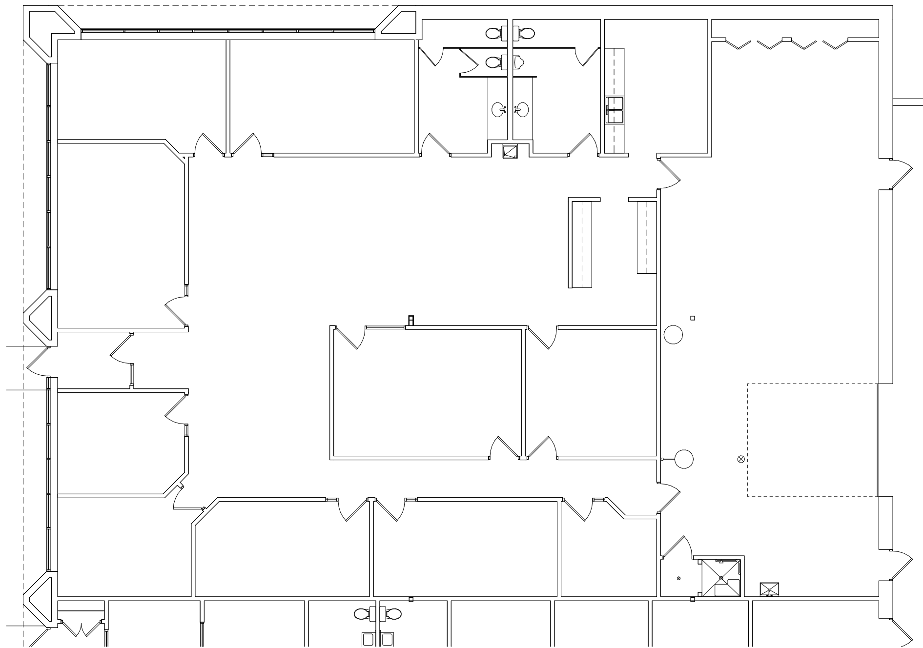
1 | Suite 100 SCALE: 1" = 10'-0"
